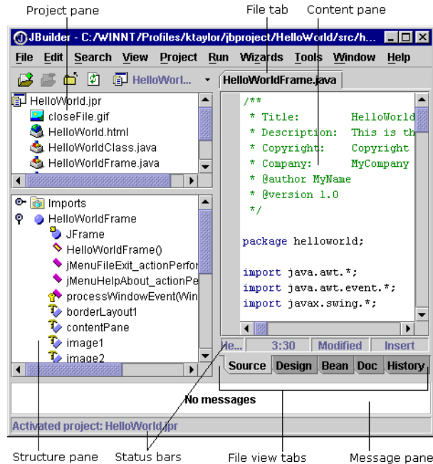
Figure 23.1 AppBrowser 요소
