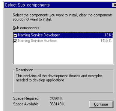
(visibrokerJava 4.gif)
