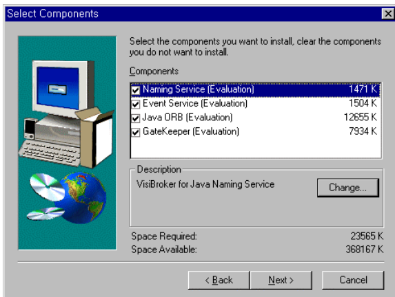
(visibrokerJava 3.gif)
