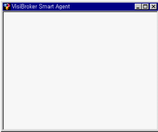
(Agent .gif)
