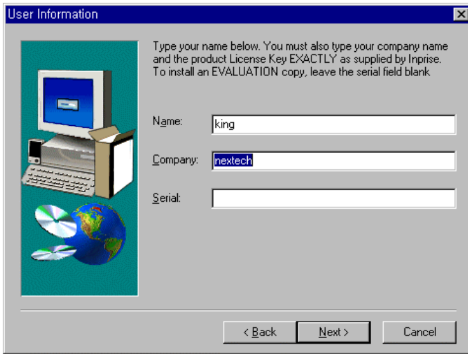
(visibrokerJava 1.gif)
