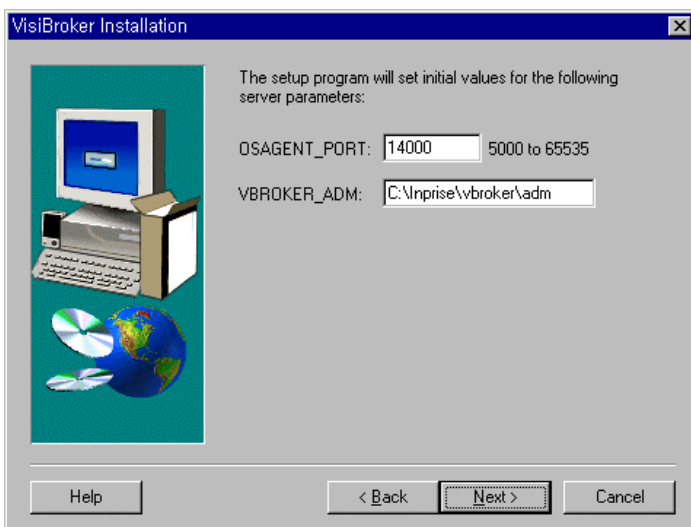
(visibrokerJava 5.gif)
