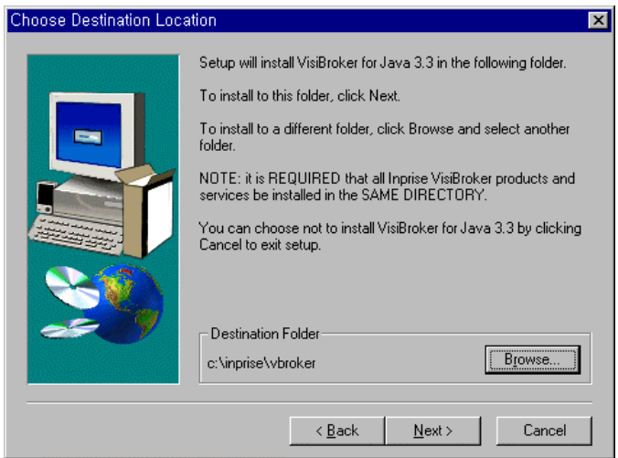
(visibrokerJava 2.gif)
