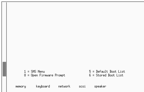
그림 2-1. SMS 콘솔
