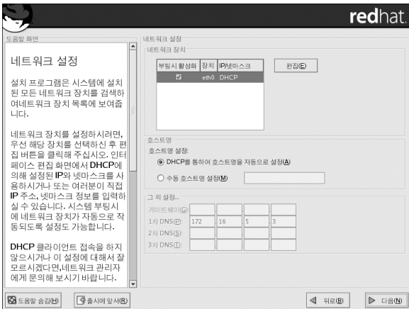
그림 2-6. 네트워크 설정
